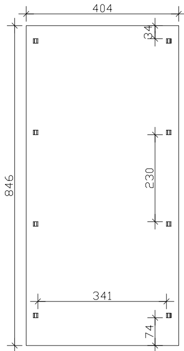
Grundriss
