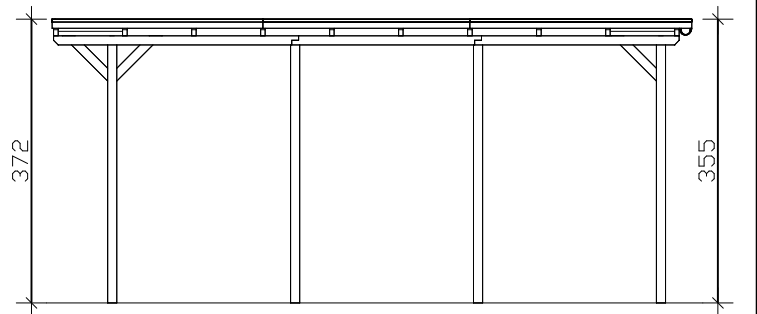
Seitenansicht
