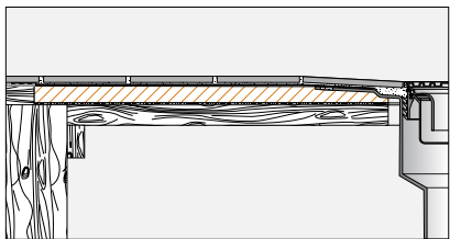
Einbaubeispiel Schlüter®-KERDI-SHOWER-TB
