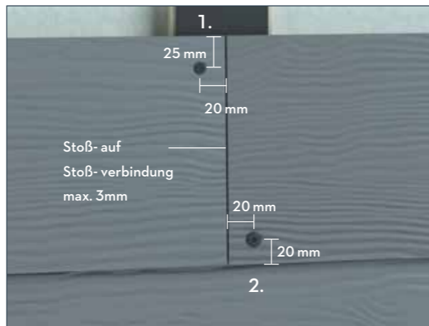
Bei Stoß-auf-Stoß-Verbindungen darauf achten, dass die aneinander stoßenden Plank nur losen Kontakt miteinander haben.
