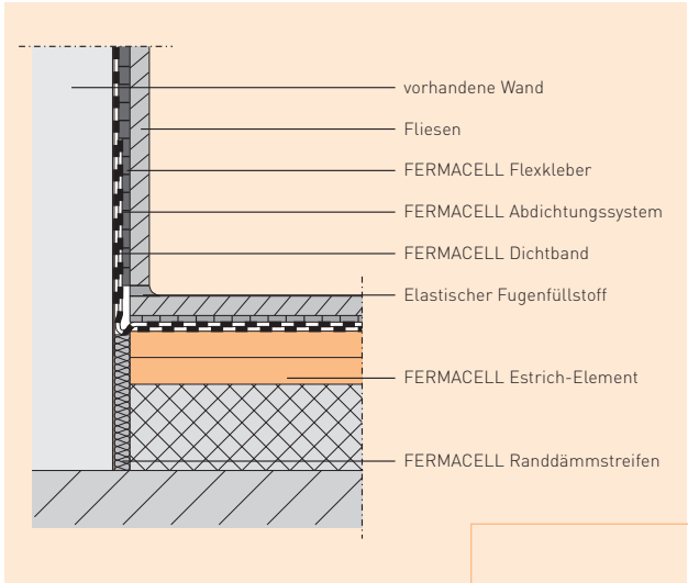
Beispiel: Wand-Fußboden-Anschluss im Wasser beanspruchten Bereich
