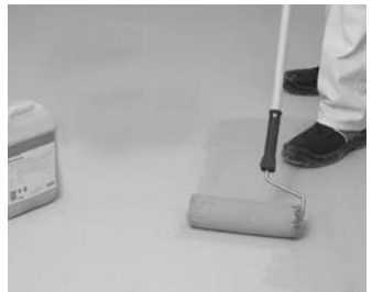
Vorbereitung: Boden grundieren und Randdämmstreifen verlegen
