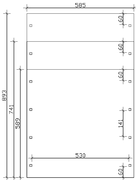
Grundriss
