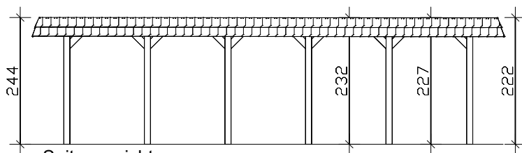
Seitenansicht
