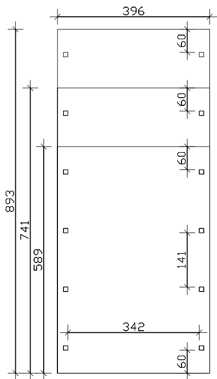
Grundriss
