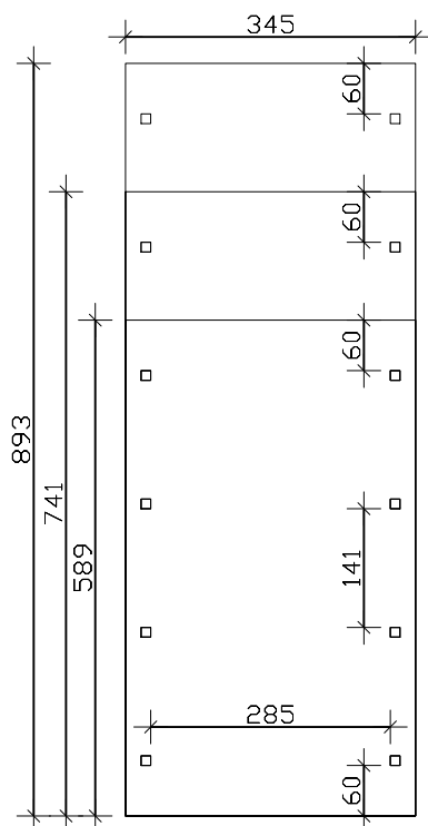
Grundriss
