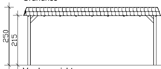
Vorderansicht
