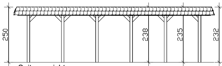
Seitenansicht
