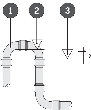
Abb. 7: Rückstauschleife
